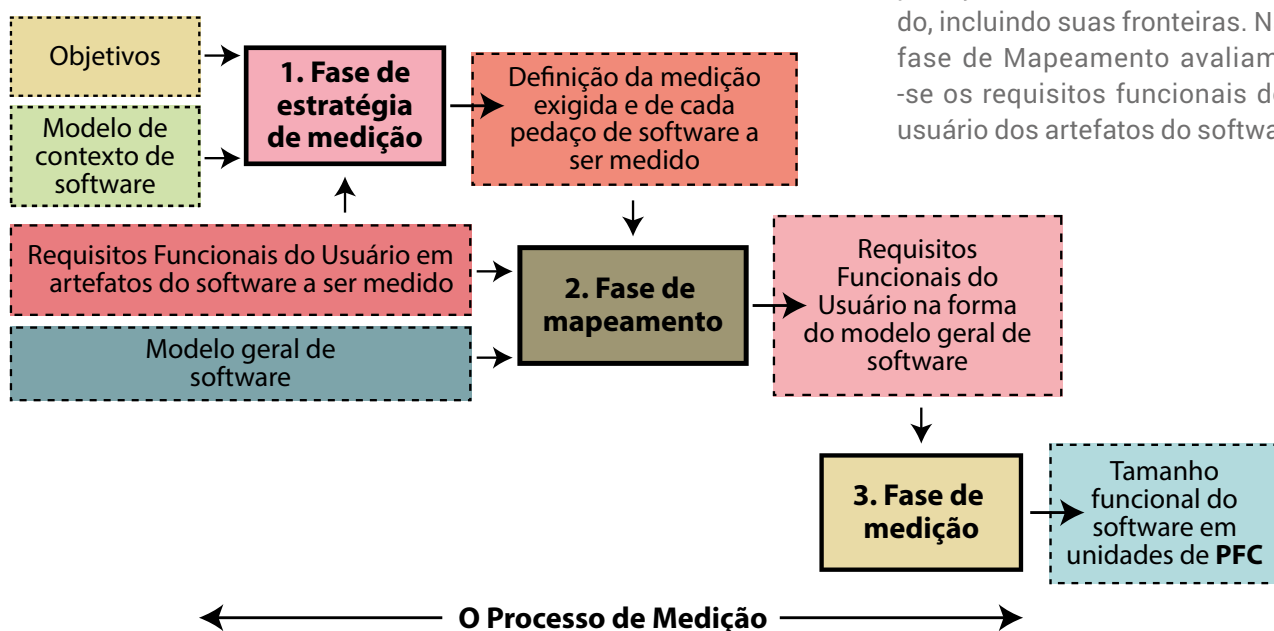
O processo de medição COSMIC
