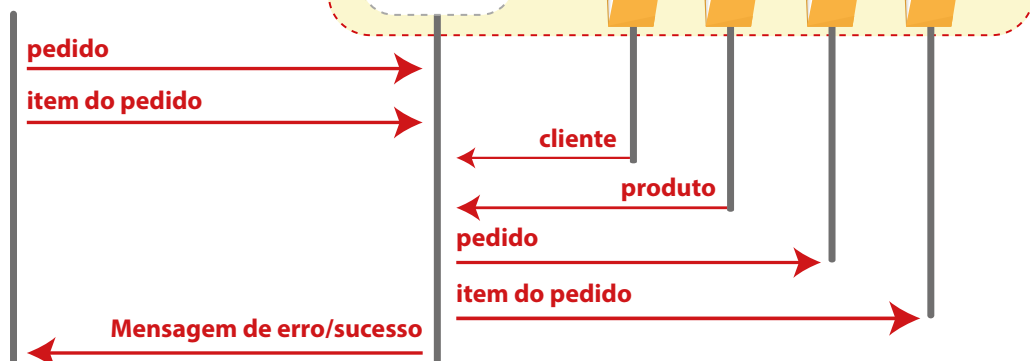
Exemplo de processo funcional com 7 movimentos de dados, ou 7 CFPs
